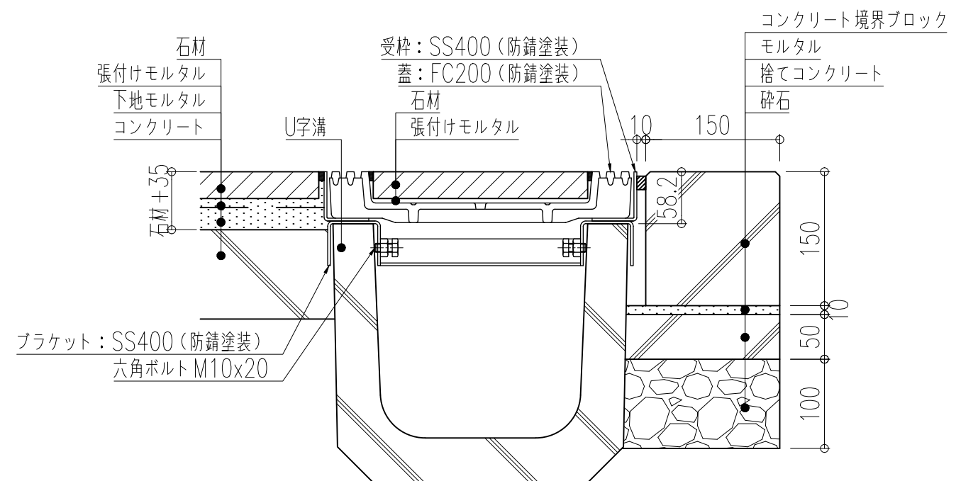
施工参考図
